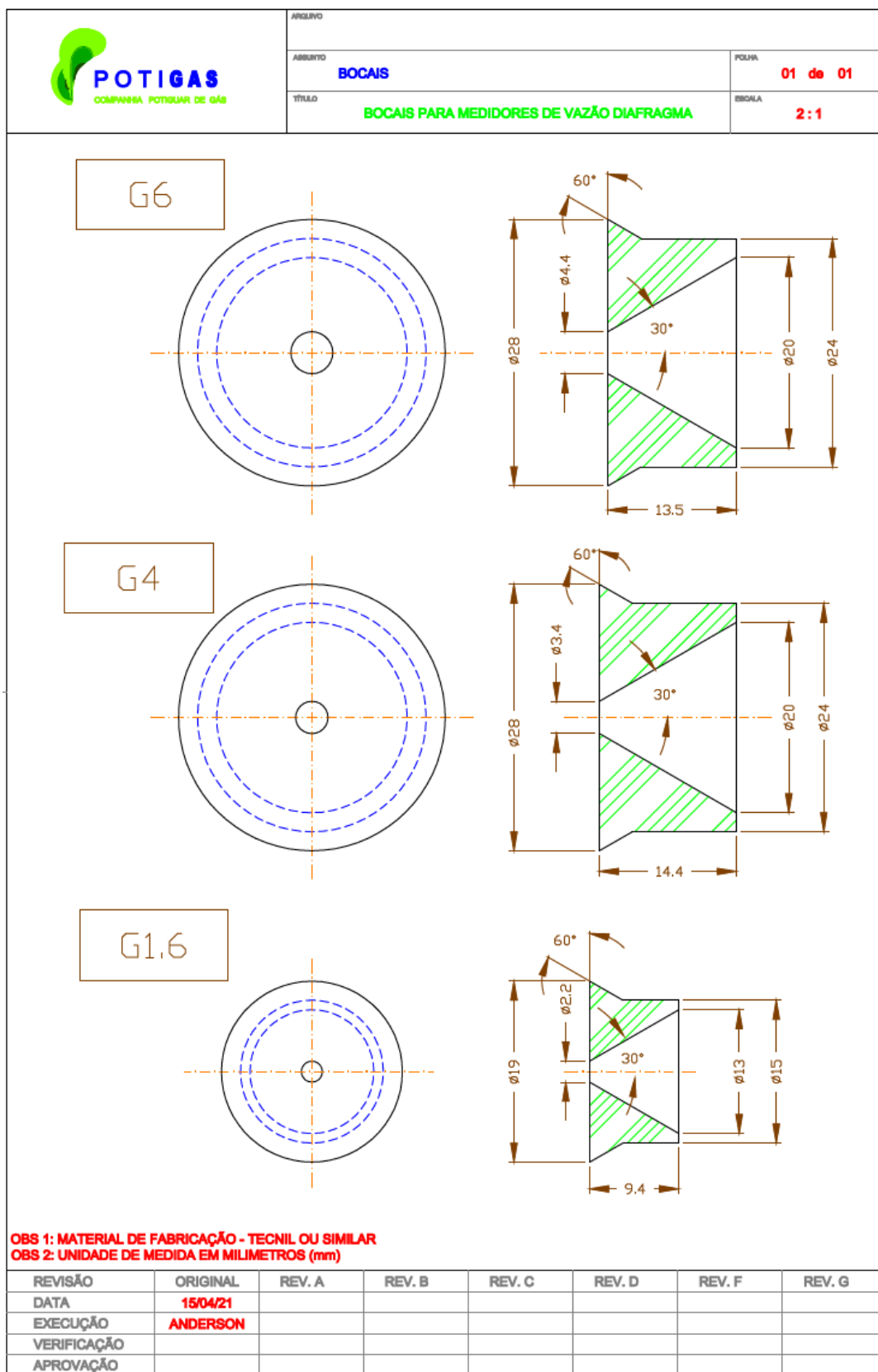
Figura 01 – Geometria dos bocais limitadores de vazão (restritores)
